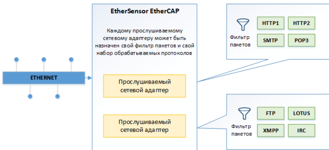
Рис.6. Варианты организации работы службы EtherSensor PCAP.
