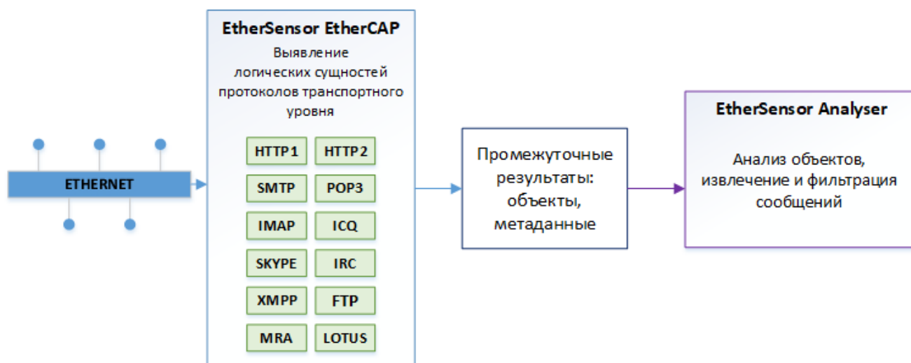
Рис.8. Схема работы службы EtherSensor EtherCAP
