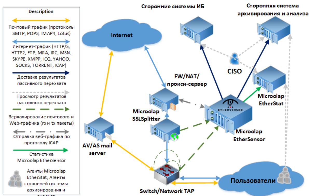
Рис.2. Типовая схема включения Microolap EtherSensor в локальной сети.
