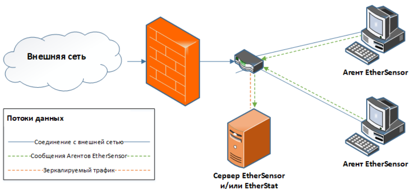
Рис.28. Прозрачное проксирование без маркировки трафика
